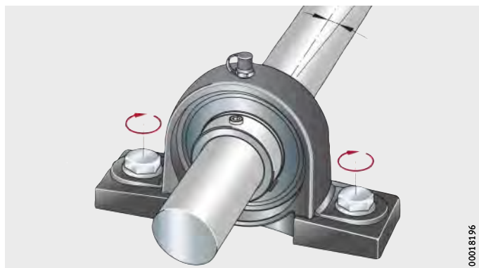
Рисунок 9 Затянуть винты крепления корпуса от руки
